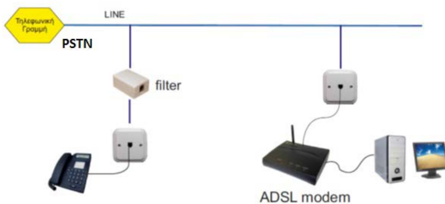
Σχήμα 5.1.4.2.β. Σύνδεση ADSL σε γραμμή PSTN με χρήση φίλτρου (splitterless) (Πηγή: http://users.sch.gr//iliaslamprou/images/stories/askiseis_electrikwn_eqkatastasewn/phones_and_lan_installation_diagram.pdf )
