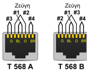
Εικόνα 2.4.1.κα: Συρμάτωση
