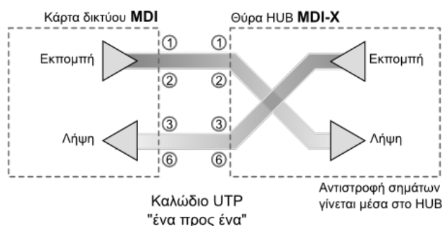
Εικόνα 2.4.3.α: MDI/MDI-X
