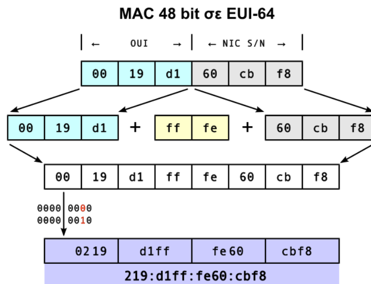
Εικόνα 3.5.1.α: Μεταγραφή διεύθυνσης MAC 48 bit σε EUI-64
