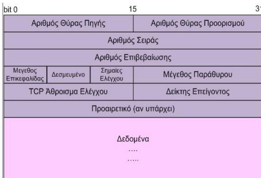
Εικόνα 4.1.1.γ: Πεδία της επικεφαλίδας ενός TCP τμήματος.
