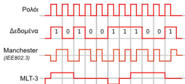
Εικόνα 2.4.1.κζ: Κωδικοποίηση Manchester, MLT-3
