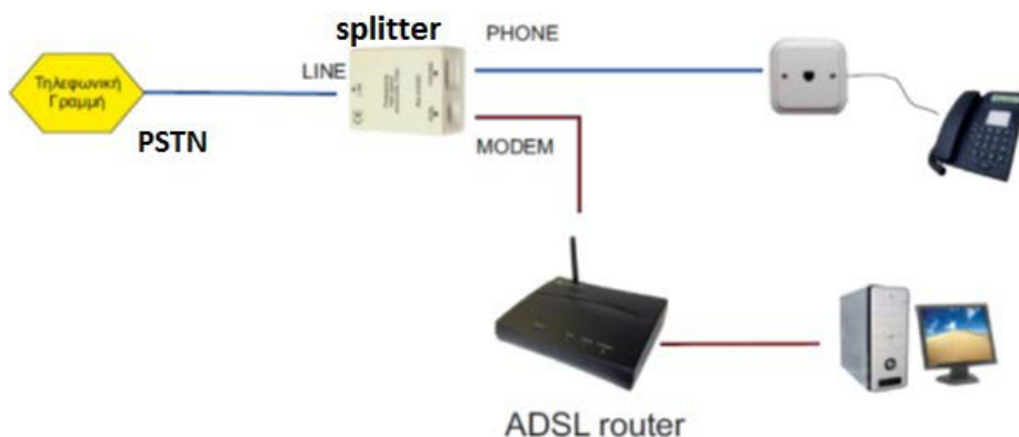
Σχήμα 5.1.4.2.γ. Σύνδεση ADSL σε γραμμή PSTN με χρήση διαχωριστή σήματος (splitter-based) (Πηγή: http://users.sch.gr//iliaslamprou/images/stories/askiseis_electrikwn_eqkatastasewn/phones_and_lan_installation_diagram.pdf )
