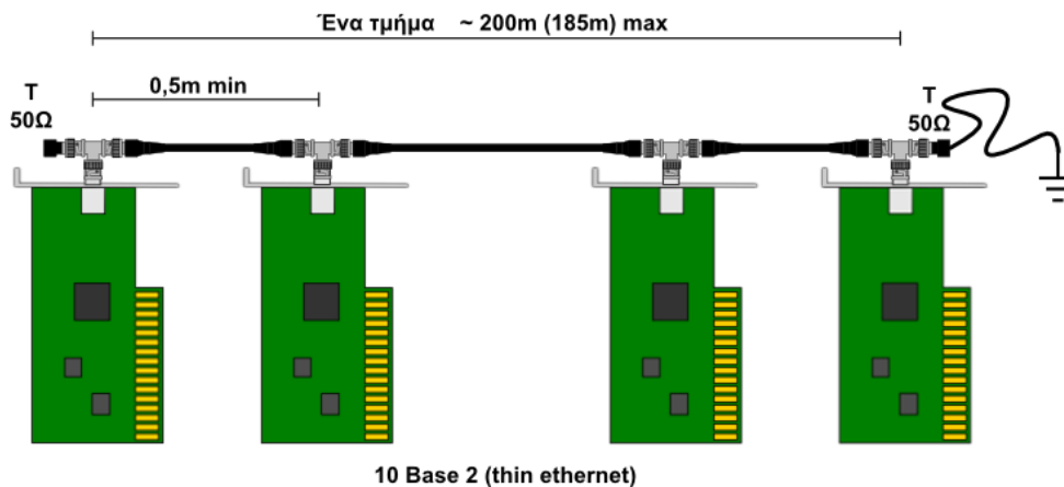
Εικόνα 2.4.1.γ: Δίκτυο Thin Ethernet (10Base2).
