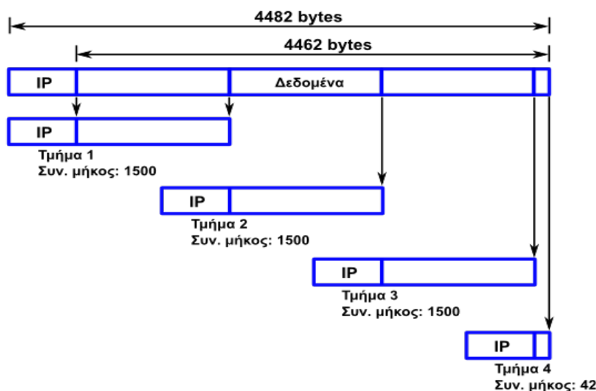
Εικόνα 3.2.γ: Κατάρτησης αυτοδύναμου πακέτου IPv4
