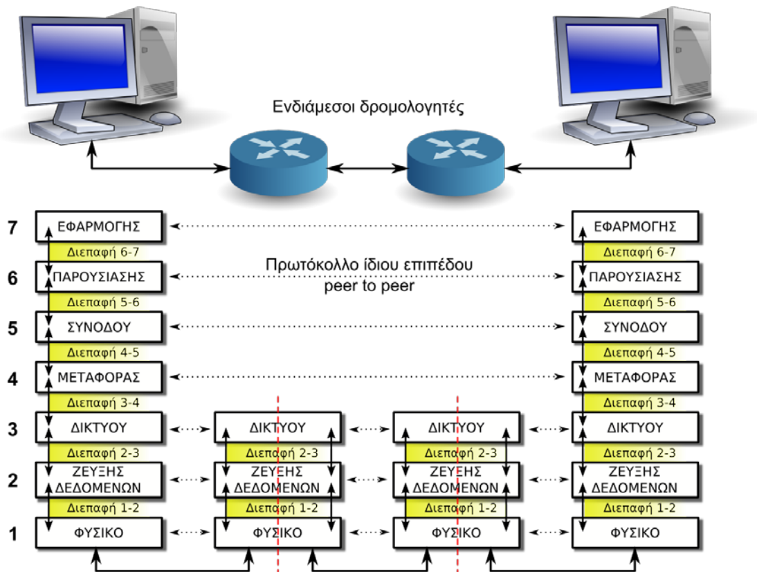
Εικόνα 1.2.1.β: Διαστρωματωμένη αρχιτεκτονική, διεπαφές και ομότιμα επίπεδα
